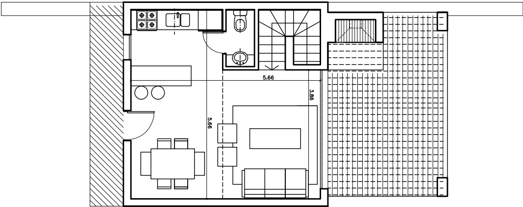
PLANTA BAJA
